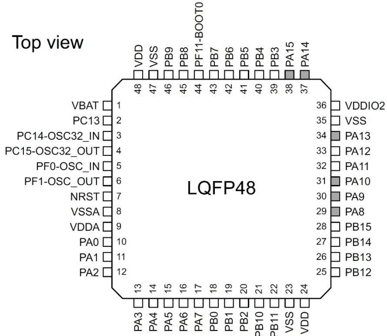
FCM32x042x LQFP48 pinout
